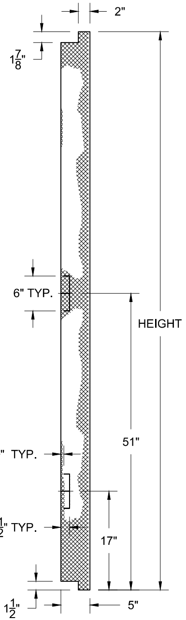
SECTION A-A
